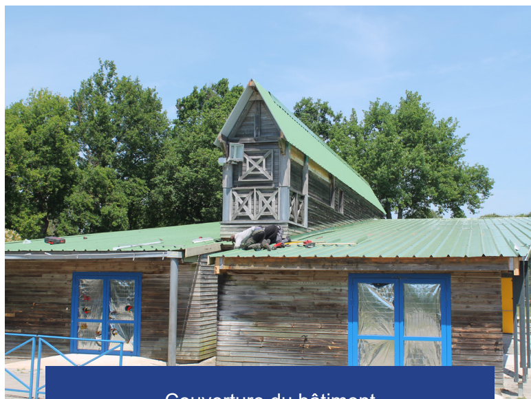
Couverture du bâtiment de la Grange aux Jeux
